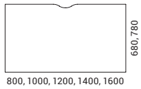
Tischplatte mit „Muschel“ Ausschnitt
